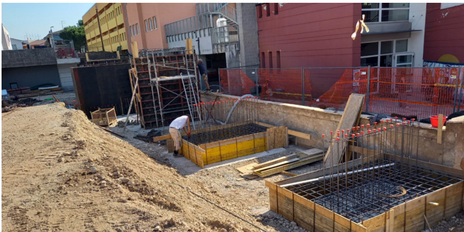
Realizzazione pile di sostegno pista ciclabile
