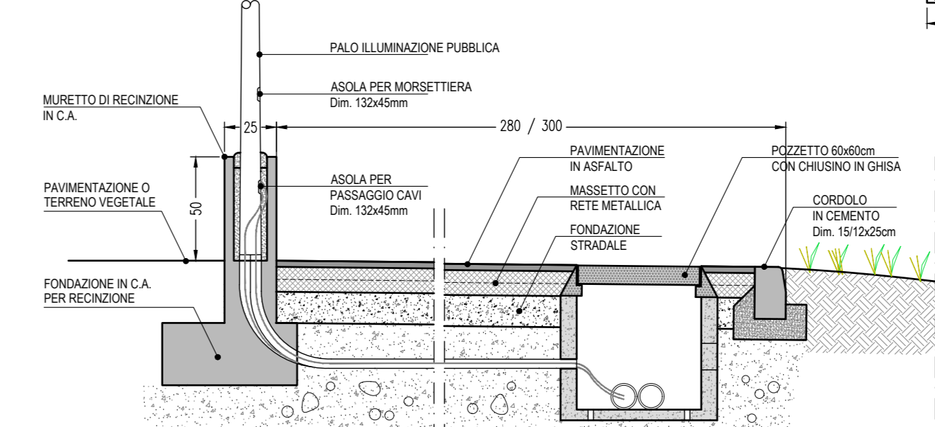
SEZIONE TIPO - PALO ILLUMINAZIONE PISTA CICLABILE scala 1:20
