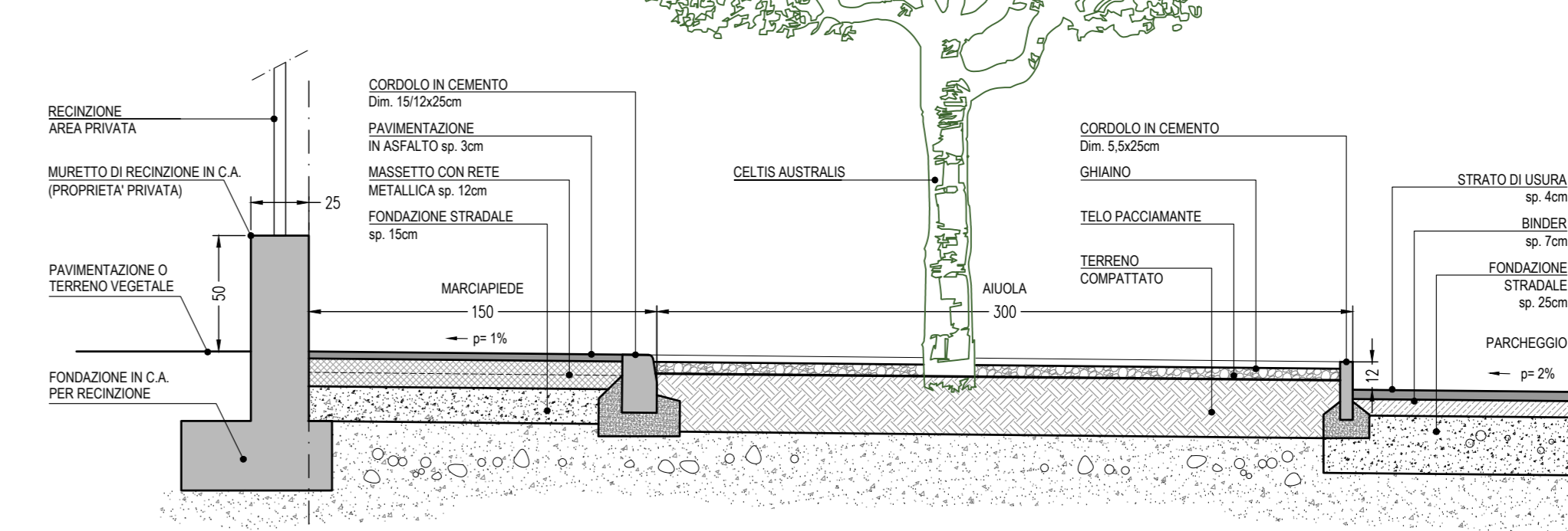
SEZIONE TIPO - AIUOLA SPARTITRAFFICO CON PALO ILLUMINAZIONE ZONA PARCHeggi VIA DELLA TECNICA (PARTICOLARE 2) scala 1:20
