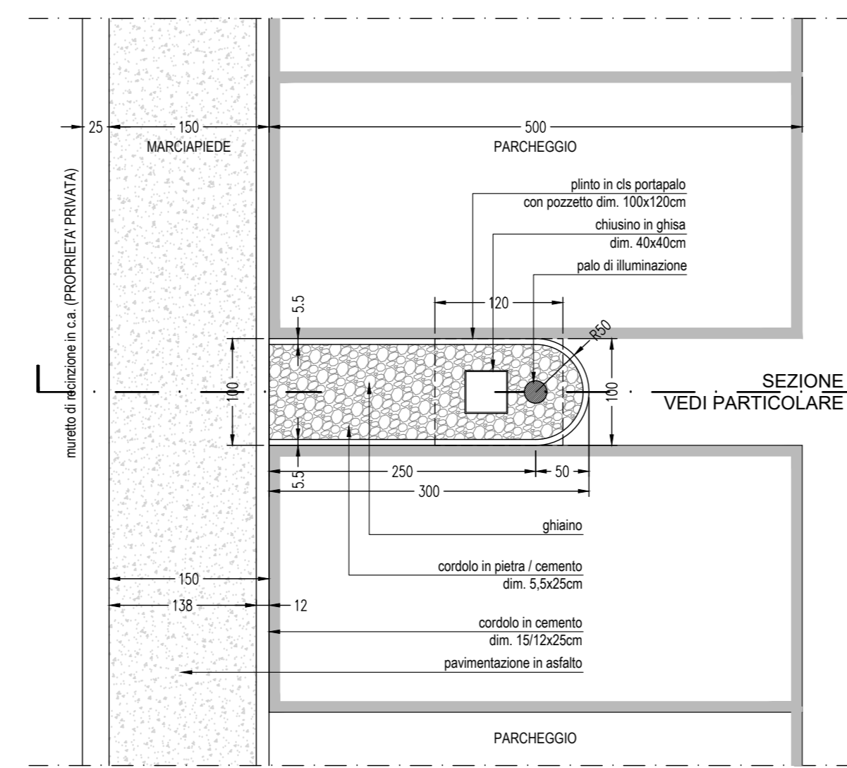
PARTICOLARE 2 - AIUOLA SPARTITRAFFICO CON PALO ILLUMINAZIONE PUBBLICA scala 1:50
