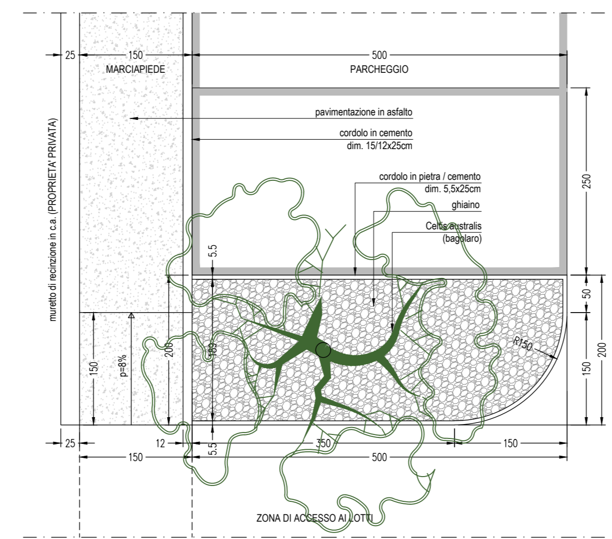
PARTICOLARE 1 - AIUOLA SPARTITRAFFICO ZONA ACCESSI AI LOTTI scala 1:50
