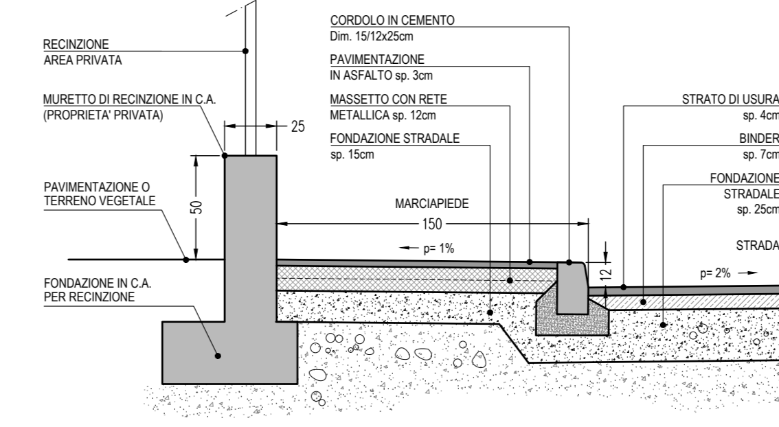
SEZIONE TIPO - MARCIAPIEDE scala 1:20
