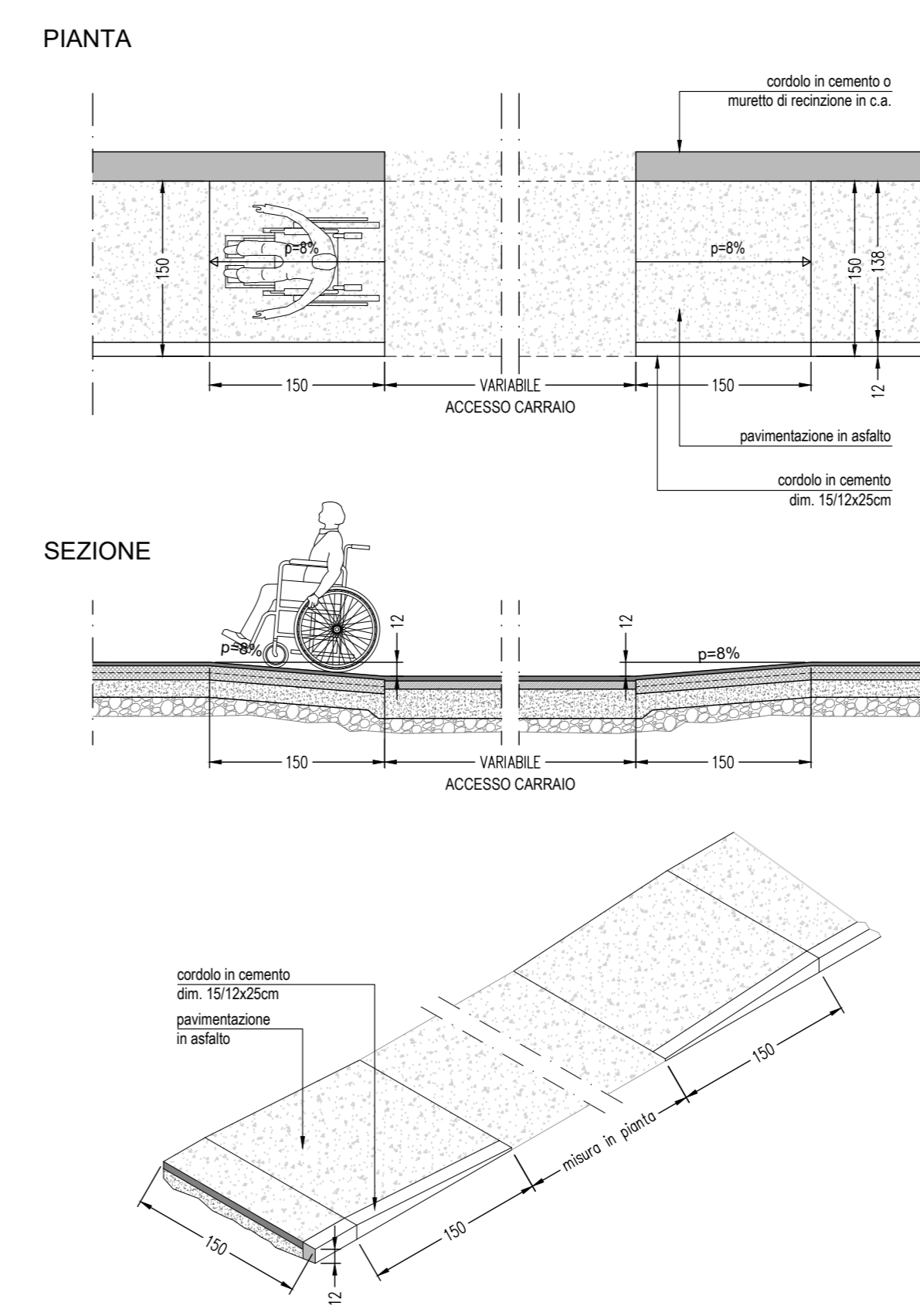
PARTICOLARE 3 - RAMPA PER DISABILI SU MARCIAPIEDI scala 1:50
