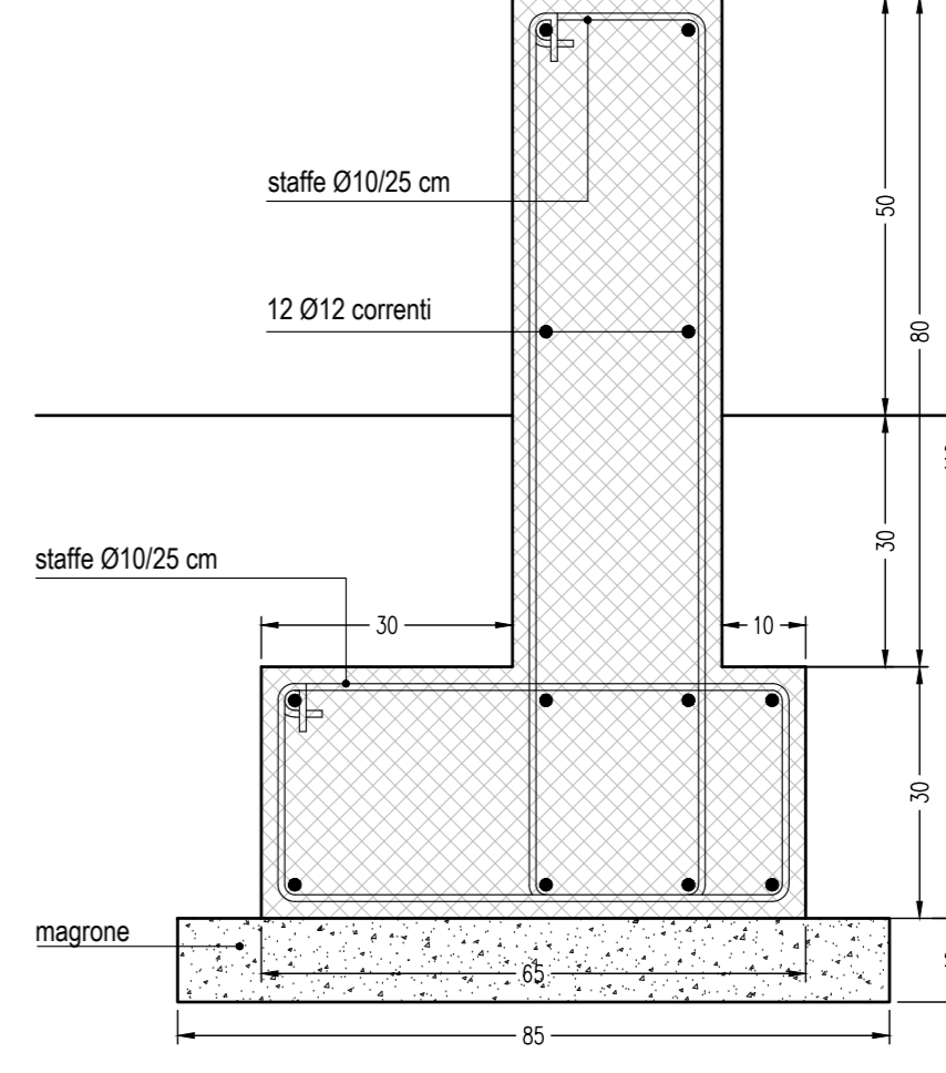
SEZIONE RECINZIONE scala 1:10
