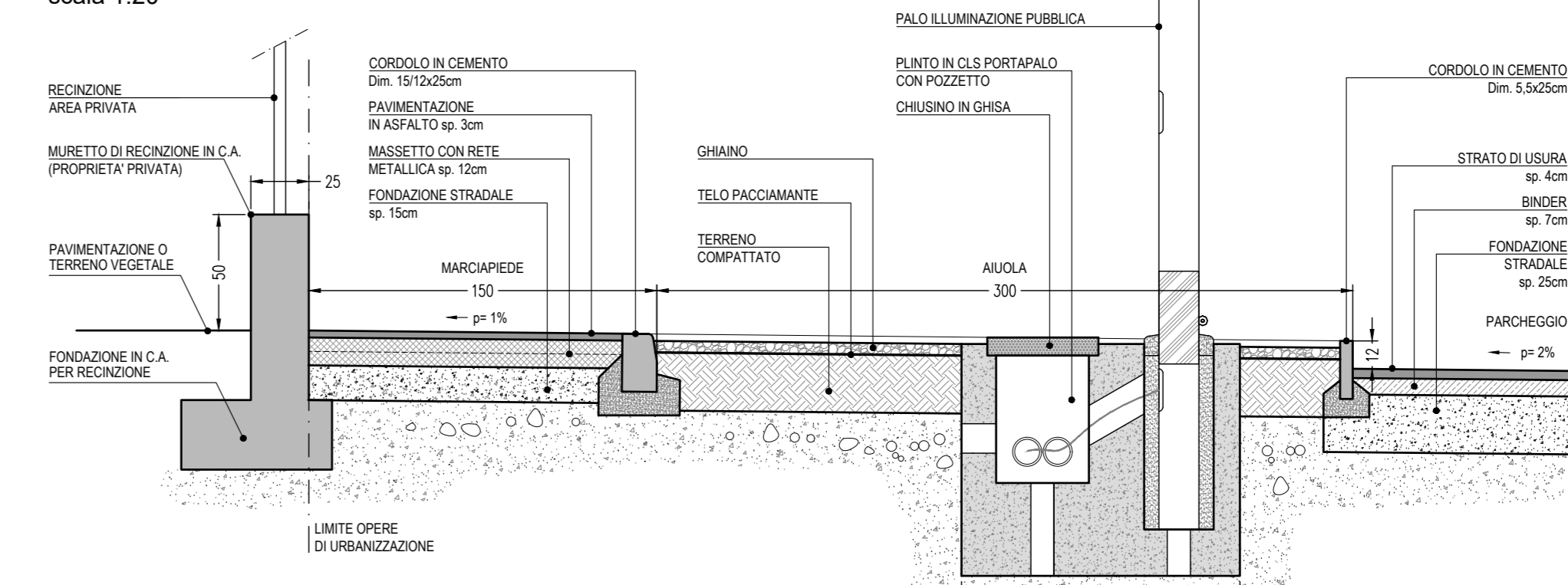
SEZIONE TIPO - AIUOLA SPARTITRAFFICO CON PALO ILLUMINAZIONE ZONA PARCHeggi VIA DELLA TECNICA (PARTICOLARE 2) scala 1:20
