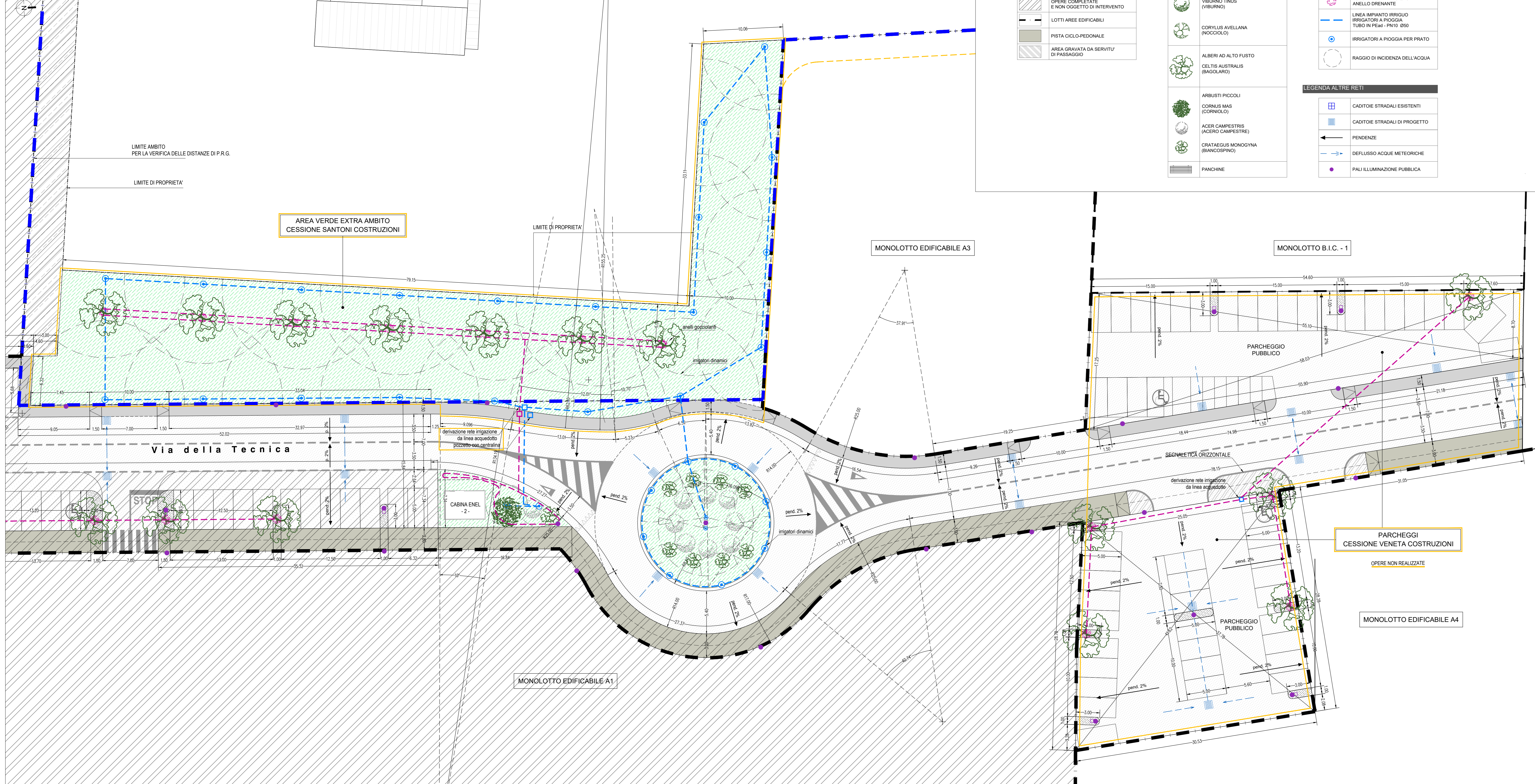
PARTICOLARE AREA VERDE E PARCHeggi TRATTO - A - VIA DELLA TECNICA scala 1:200
