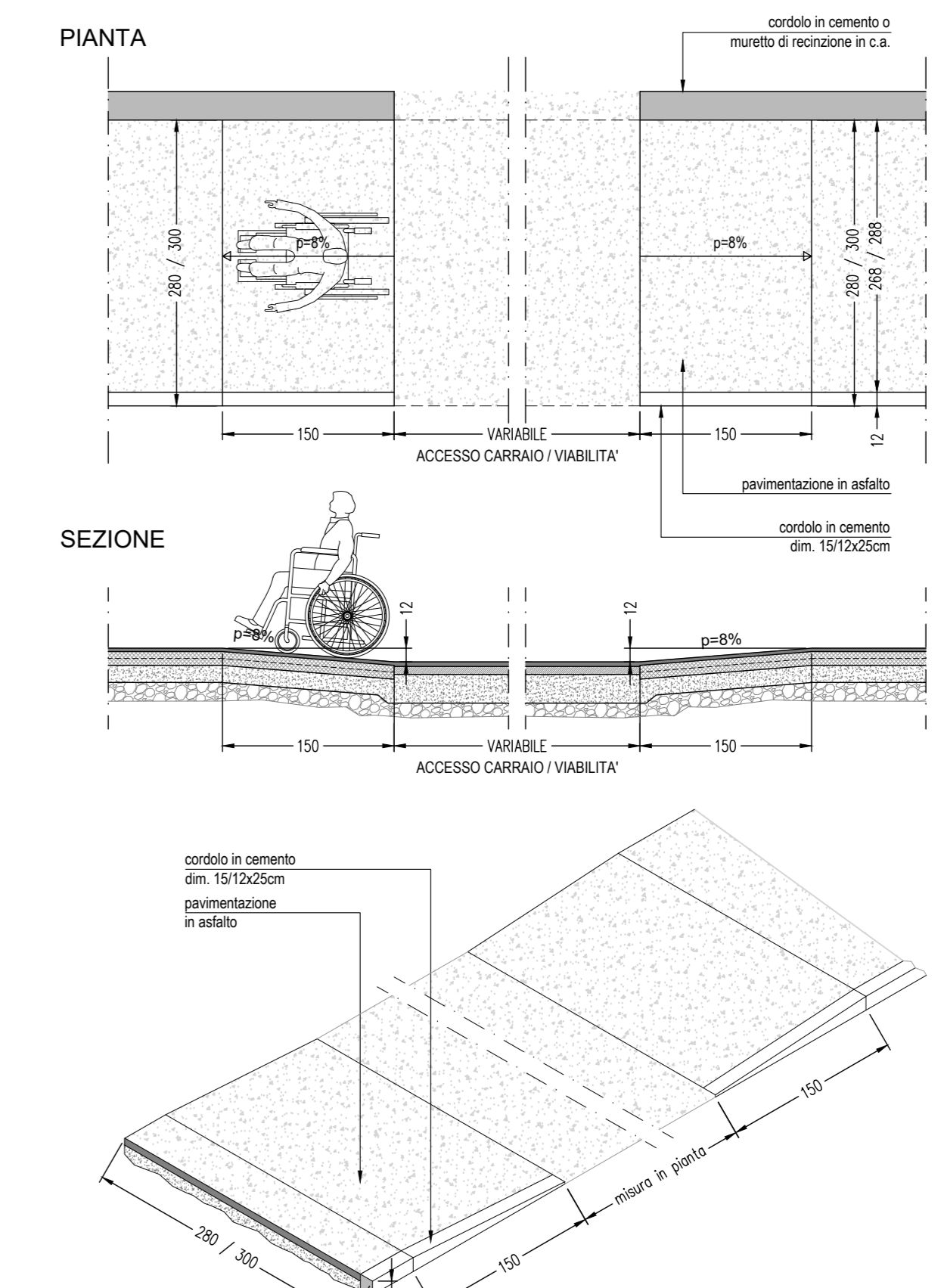
PARTICOLARE 4 - RAMPA PER DISABILI SU PISTA CICLOPEDONALE scala 1:50
