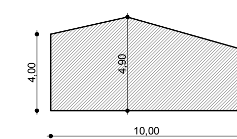
sezione E-E
