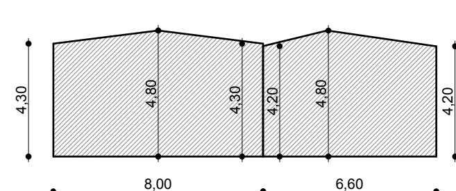
sezione B-B
