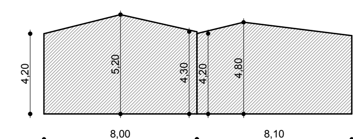
sezione C-C
